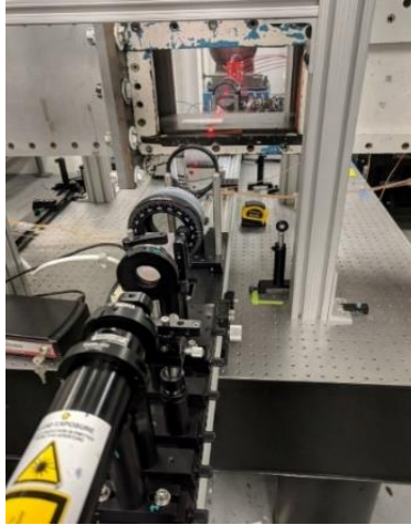
Figure 2 : Exemple de montage en veine proposé par [4]
