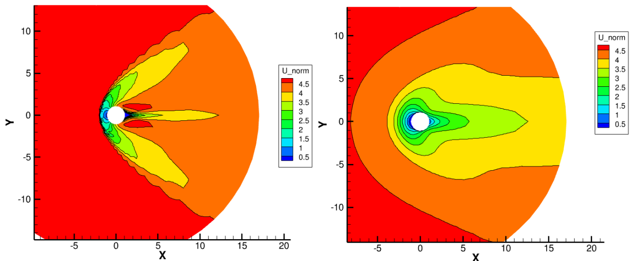
Fig.1 : Simulation UGKS d'un écoulement d'Argon à Mach 5 autour d'un cylindre. A gauche : Kn = 10^{-4} . A droite : Kn = 1 .
