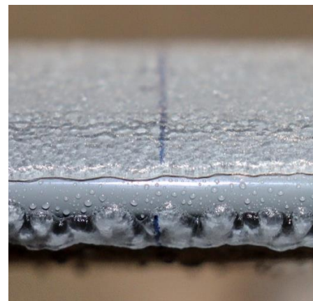
Figure 2: profil avec formation de givre et bord d'attaque anti-givré (image tirée de [1])
