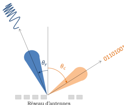
Figure 1 : Système MIMO DFRC. Les formes d'ondes se recombinaient en un signal radar dans la direction \theta_r , et un signal de communication dans la direction \theta_c .
