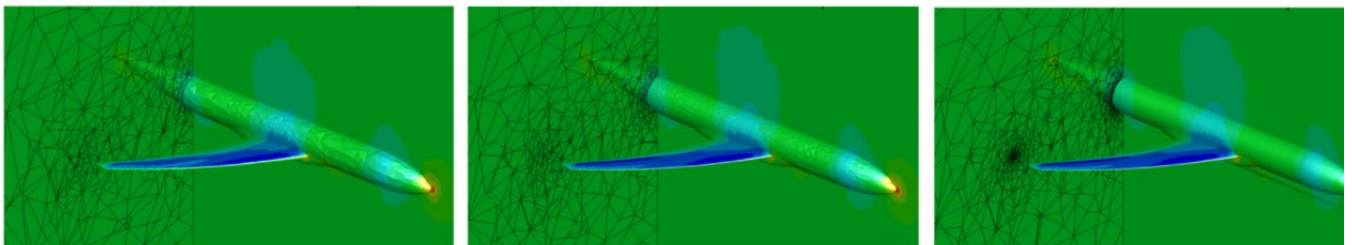
Figure: Adaptations en maillage isotrope successives d'une configuration d'avion CRM, F. Basile 2022 [5]
