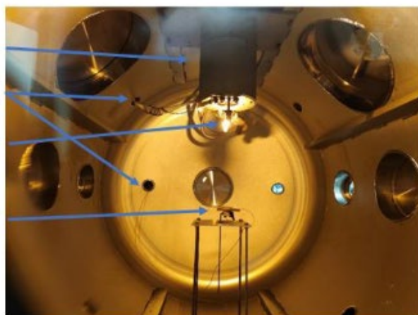
Figure 1 Source plasma en fonctionnement dans PICOMAX-E
