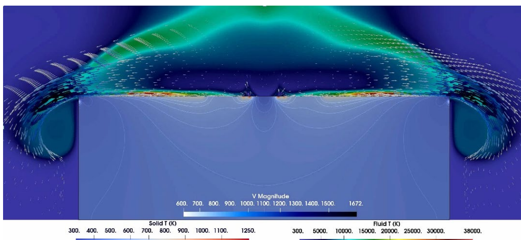
Figure 1- Champs de température et de vitesse dans simulation numérique de chambre à arc couplé à la dégradation de l'électrode, réalisée avec le code MoDeTheC avec l'aide d'une méthode de Super-Timestepping.
